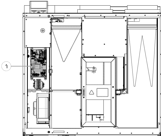
Joon. 7. Trükkplaadi asend
