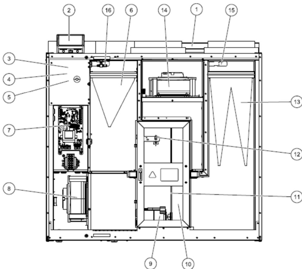
Joon. 10. Sisemised komponendid
