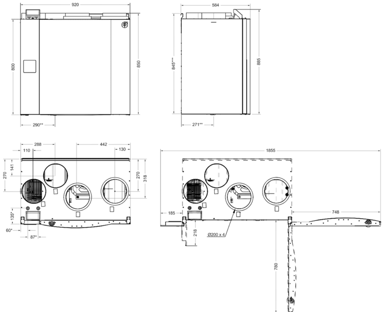
Joonis 1. Mõõdud ja kaal, L-mudel
