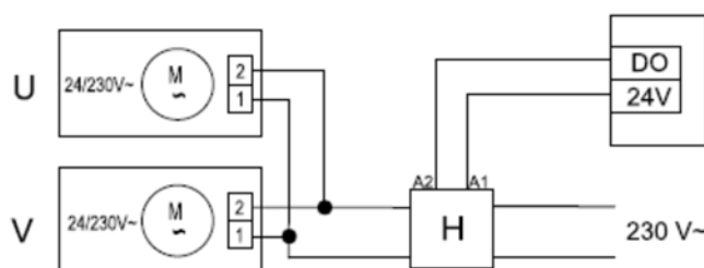
Joonis 18. Klapiühendus
