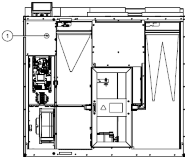
Joon 11. Ülekuumenemiskaitse lähtestamise nupp
