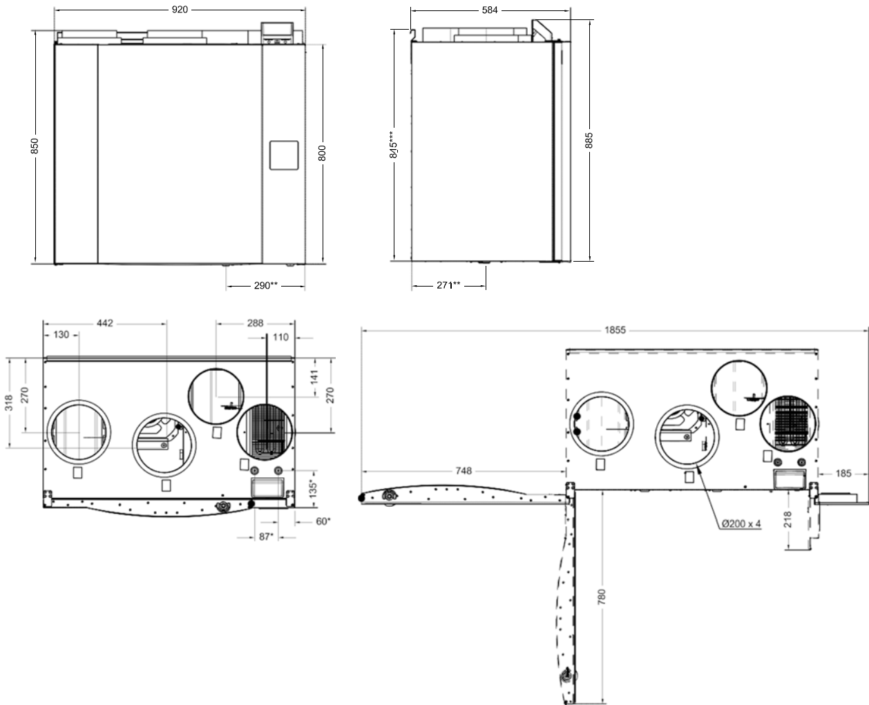
Joonis 2. Mõõdud ja kaal, R-mudel
