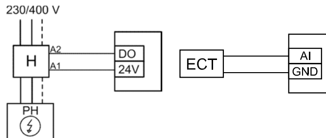
Joonis 13. Eelsoojendi ühendused
