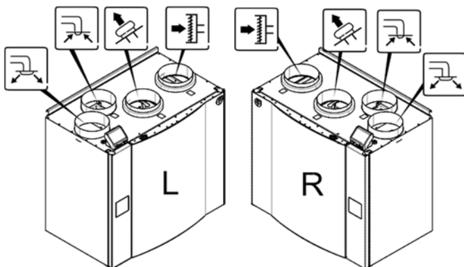
Joonis 3. Õhukanalite ühendused
